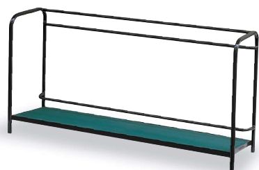
17 スチールパイプバッグ立て 1800×500×900mm スチール製 色: 黒 底面: ゴム製 色: 緑 重量 約17kg 片面フリータイプ
