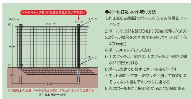
986 落球防止ネット ネット:1.2×50m 化繊製 色:茶 ボール:25.4Φ×1500mm スチール製 色:茶 16本入 キャップ:26Φmm 樹脂製 色:茶 16個入 ネット取付フック16セット付 986-1 落球防止用ネットのみ 巾1m以上 化繊製 色:茶 986-2 落球防止用ネットのみ 巾1m未満 化繊製 色:茶
