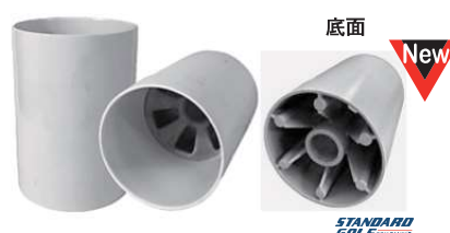
501-J アルミホールカップ 108φ×115mm アルミ製 耐久性に優れたホールカップです。カップの底に6つの足があり沈み込みを防ぐため、メンテナンスも簡単です。
