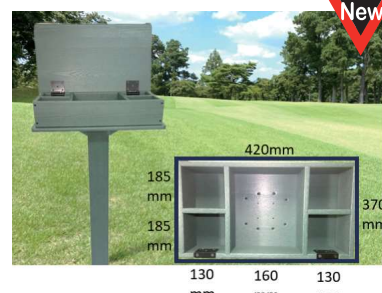
703 スコアカードキャディ 本体:420×370×12.5Hmm 再生プラスチック製 足:10×10×1200mm 樹脂製 色:緑 ティグラウンドに設置できるスコアカード入れ となります。再生プラスチックのため、錆びにくく、 メンテナンスもしやすくなっております。
