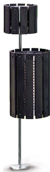
336-S 灰皿くずかご スタンド ウッド製 (埋込金具付) (上)180Φ×150mm 4ℓ 木製 (下)220Φ×350mm 13ℓ 木製 全長900mm 灰皿:ステンレス製 色:茶
