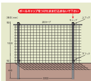
986 落球防止ネット ネット:1.2×50m 化繊製 色:茶 ポール:25.4φ×1500mm スチール製 色:茶 16本入 キャップ:26φmm 樹脂製 色:茶 16個入 ネット取付フック16セット付
