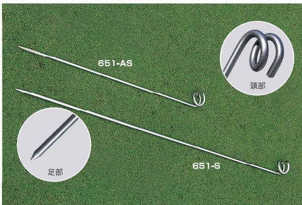
651-AS ステンレス ロープ止棒 (小) 8Φ×600mm ステンレス製
