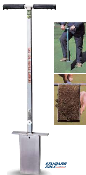
517-A ソイルテスター(大) 95×200×20t mm スチール製 深さ20cm、幅10cm、厚さ2cmの土壤 サンプルを抽出できます。面でサンプ ルを採取するため、細かく芝生の根の 確認を行うことができます。
