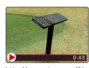
702 擬木ティホルダー 天板:660×200×30t mm 擬木製 杭:80φ×1000mm 擬木製 ショートホールのティーイングエリアに設置して、ショートティをサービスするためのホルダーです。
