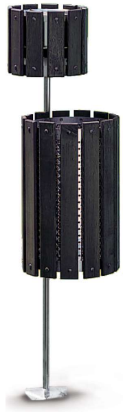
336-S 灰皿くずかご スタンド ウッド製 (埋込金具付) (上) 180Φ×150mm 4ℓ (下) 220Φ×350mm 13ℓ 全長900mm 灰皿: ステンレス製 色: 茶
