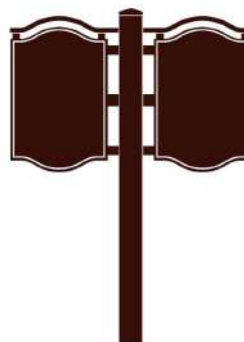
489-B-1-0 489B2枚表示指示板 板:600×400×20mm アルミ製 文字板:シート加工 片面表示 色:茶 足:130×130×2000mm 擬木製スチール芯入り 色:茶 アルミ製の2枚表示の指示板です。文字板はシート加工のため、ご要望に応じたデザインが可能です。支柱は擬木製角柱です。コースの案内板やヤード表示板など様々にご利用いただける高級感のある案内指示板です。 →P59
