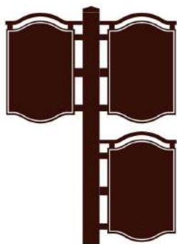
489-B-2-0 489B3枚表示指示板 板:600×400×20mm アルミ製 文字板:シート加工 片面表示 色:茶 足:130×130×2000mm 擬木製スチール芯入り 色:茶 アルミ製の3枚表示の指示板です。文字板はシート加工のため、ご要望に応じたデザインが可能です。支柱は擬木製角柱です。コースの案内板やヤード表示板など様々にご利用いただける高級感のある案内指示板です。 →P59
