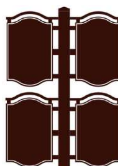
489-B-3-0 489B4枚表示指示板 板:600×400×20mm アルミ製 文字板:シート加工 片面表示 色:茶 足:130×130×2000mm 擬木製スチール芯入り 色:茶 アルミ製の4枚表示の指示板です。文字板はシート加工のため、ご要望に応じたデザインが可能です。支柱は擬木製角柱です。コースの案内板やヤード表示板など様々にご利用いただける高級感のある案内指示板です。 →P59
