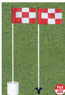
503-RW 米国式練習グリーン用マーカー フラッグ:240×160mm ナイロン製 赤白 ポール:830mm グラスファイバー製 白 カップ:108Φ×100mm 受け皿:92Φmm 樹脂製 黒
