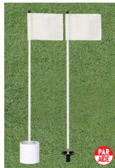
503-W 米国式練習グリーン用マーカー フラッグ:240×160mm ナイロン製 白 ポール:830mm グラスファイバー製 白 カップ:108Φ×100mm 受け皿:92Φmm 樹脂製 黒
