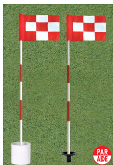
503-E 米国式練習グリーン用マーカー フラッグ:240×160mm ナイロン製 赤白 ポール:830mm グラスファイバー製 赤白 カップ:108Φ×100mm 受け皿:92Φmm 樹脂製 黒
