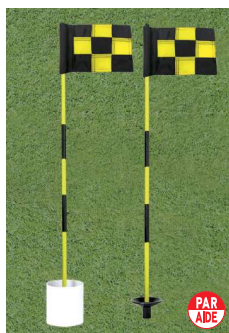
503-I 米国式練習グリーン用マーカー フラッグ:240×160mm ナイロン製 黄黒 ポール:830mm グラスファイバー製 黄黒 カップ:108Φ×100mm 受け皿:92Φmm 樹脂製 黒
