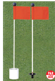
503-C 米国式練習グリーン用マーカー(ヘッド付) ヘッド:44.5Φmm 樹脂製 黒 フラッグ:240×160mm ナイロン製 赤、白、黄 ボール:830mm グラスファイバー製 白 カップ:108Φ×100mm 受け皿:92Φmm 樹脂製 黒
