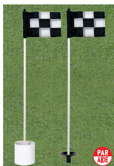
503-B 米国式練習グリーン用マーカー フラッグ:240×160mm ナイロン製 黒白 ポール:830mm グラスファイバー製 白 カップ:108Φ×100mm 受け皿:92Φmm 樹脂製 黒
