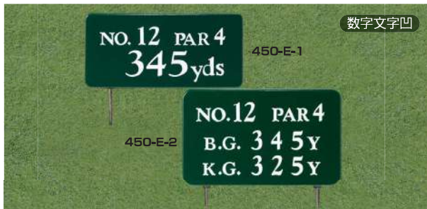
450-E-1 ヤード板 ワングリーン表示 200×400×18mm 凹表示 250mmステンレス製足
