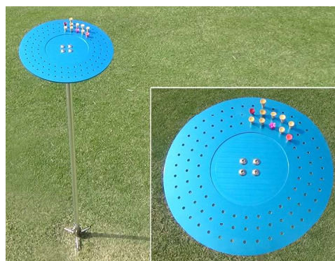
702-A 可動式ティホルダー ヘッド:300φ×高さ1000mm 支柱部:アルミ製 足部:ステンレス製 ショートホールのティーイングエリアに設置し、ショートティをプレイヤーにサービスするためのホルダーです。 可動式のため、設置しないときは取り外しが簡単です。
