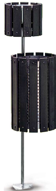
336-S 灰皿くずかご スタンド ウッド製 (埋込金具付) (上)180Φ×150mm 4ℓ (下)220Φ×350mm 13ℓ 全長900mm 灰皿:ステンレス製
