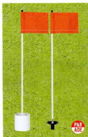
503-A フラッグ: 240×160mm ナイロン製 ポール: 830mm グラスファイバー製 カップ: 108Φ×108mm プラスチック製
