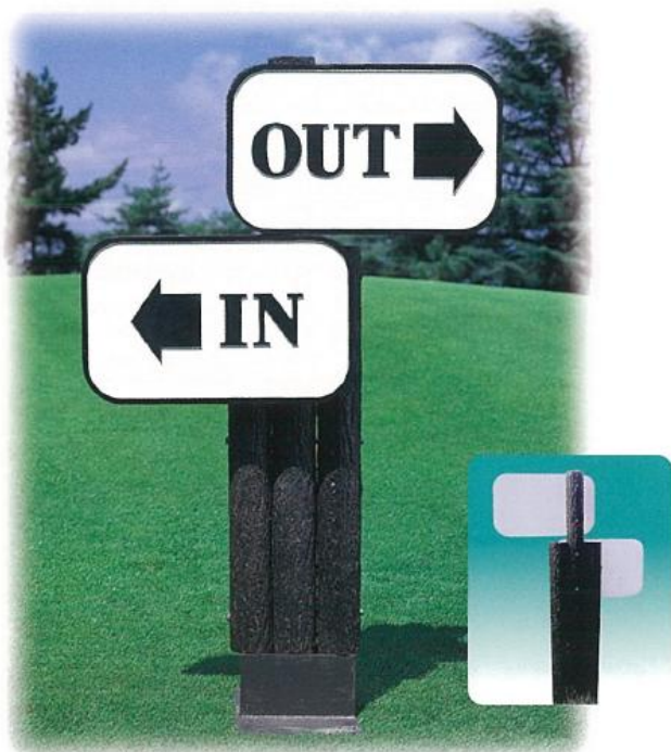
489-A 擬木コース指示板 IN-OUT板寸法 370×600mm アルミ製 擬木部 100φ×1500mm 3本組
