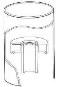
500-C ホールカップ ステンレス製 108φ×160Hmm ステンレス発音板付
